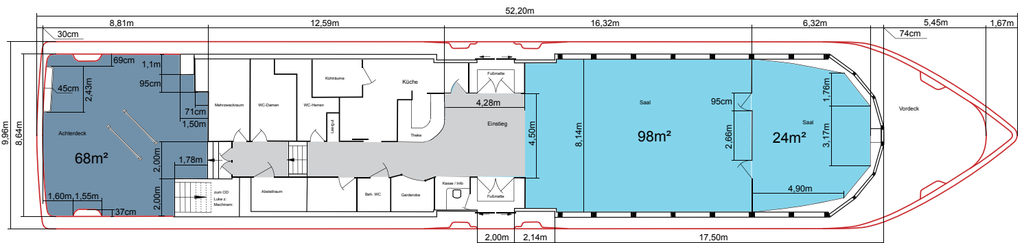
Hauptdeck
