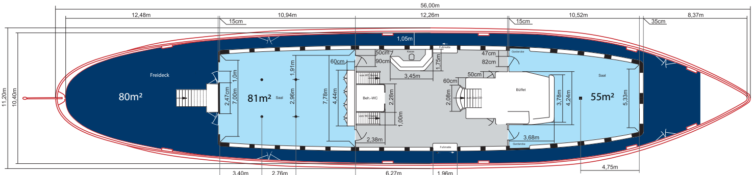
Hauptdeck
