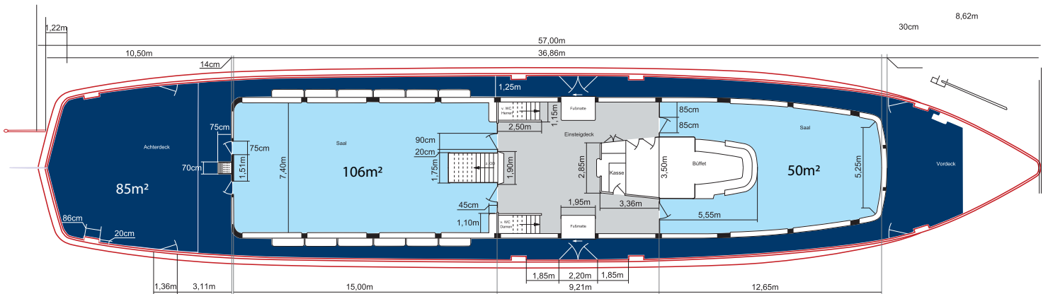
Hauptdeck
